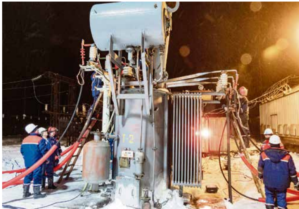
Замена трансформатора на подстанции 604
